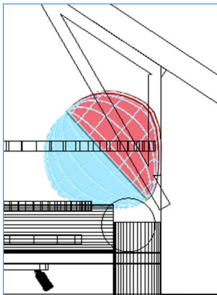
Εικόνα 6: Θέση ταινίας LED σε σχέση με τον τοίχο και τον αεραγωγό
