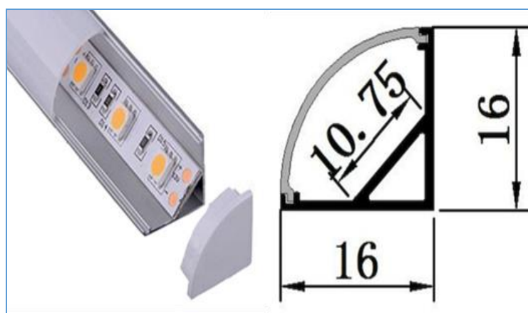
Εικόνα 5: Ενδεικτικό προφίλ αλουμινίου με διαστάσεις
